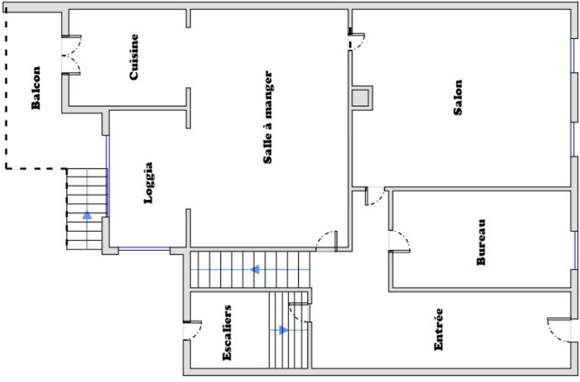
Demi niveau sur escalier jardin
