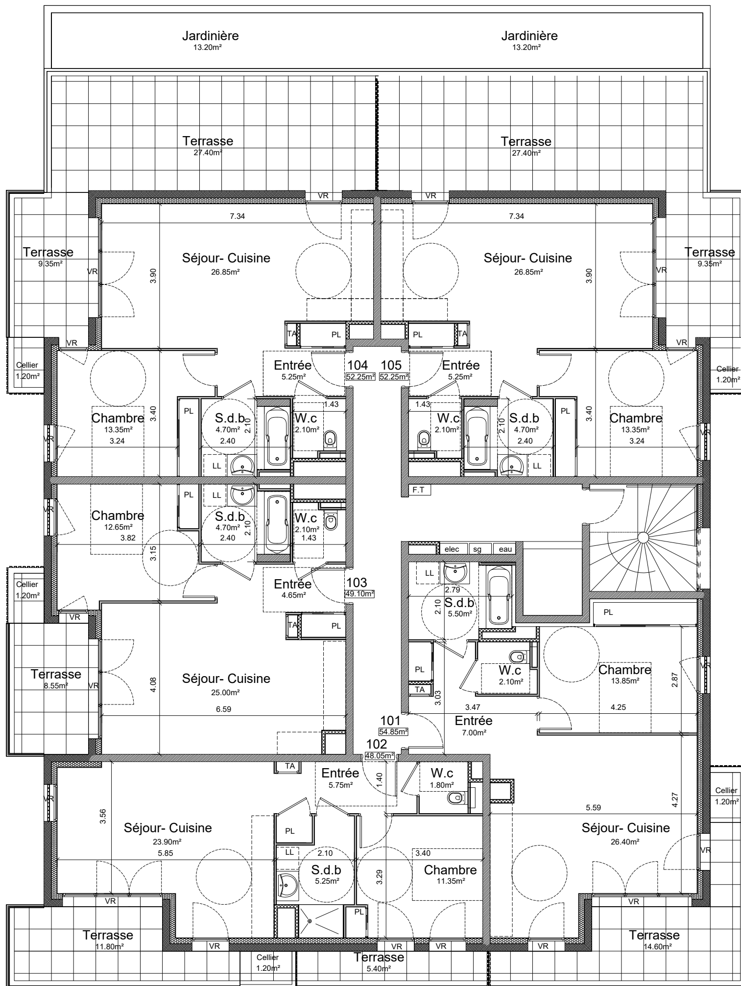
Etage 1 ech : 1/100
