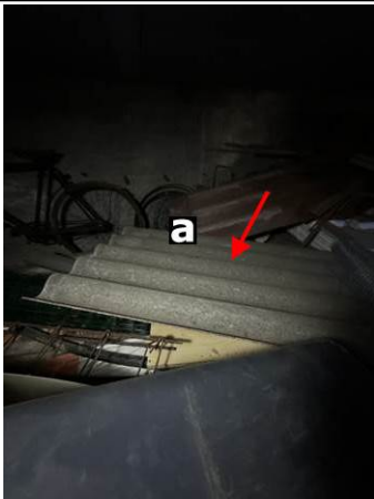
Photo n° PhA004 Localisation : Vide sanitaire Ouvrage : 1 - Couvertures, Toitures, Terrasses et étanchéités - Plaques ondulées et planes Partie d'ouvrage : Plaques en fibres-ciment (y compris plaques « sous tuiles ») Description : Plaques en fibres-ciment (y compris plaques « sous tuiles ») Localisation sur croquis : M004
