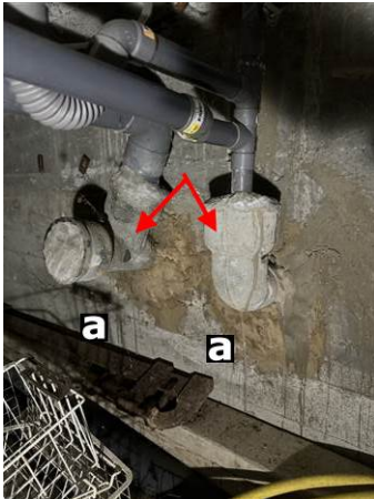
Photo n° PhA002 Localisation : Vide sanitaire Ouvrage : 6 - Conduits et accessoires intérieurs - Conduits de fluides (air, eau, vapeur, fumée, échappement, autres fluides) Partie d'ouvrage : Conduit en fibres-ciment Description : Conduit en fibres-ciment Localisation sur croquis : M002
