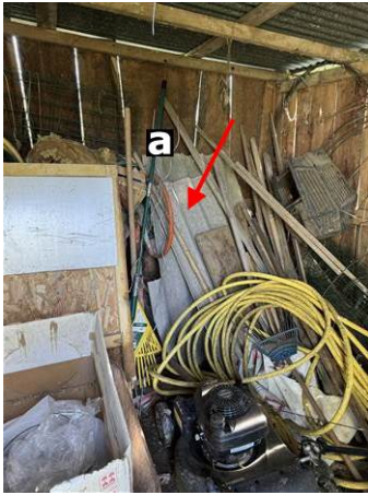
Photo n° PhA001 Localisation : Abri 2 Ouvrage : 1 - Couvertures, Toitures, Terrasses et étanchéités - Plaques ondulées et planes Partie d'ouvrage : Plaques en fibres-ciment (y compris plaques « sous tuiles ») Description : Plaques en fibres-ciment (y compris plaques « sous tuiles ») Localisation sur croquis : M001
